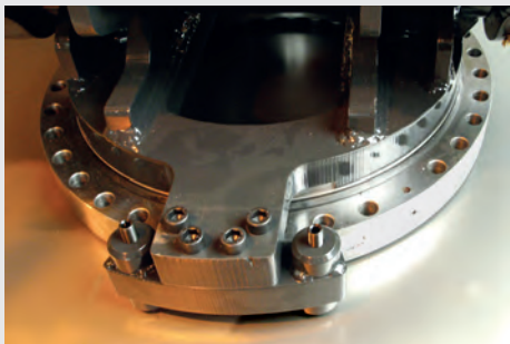
Schwenkbremse slewing brake
